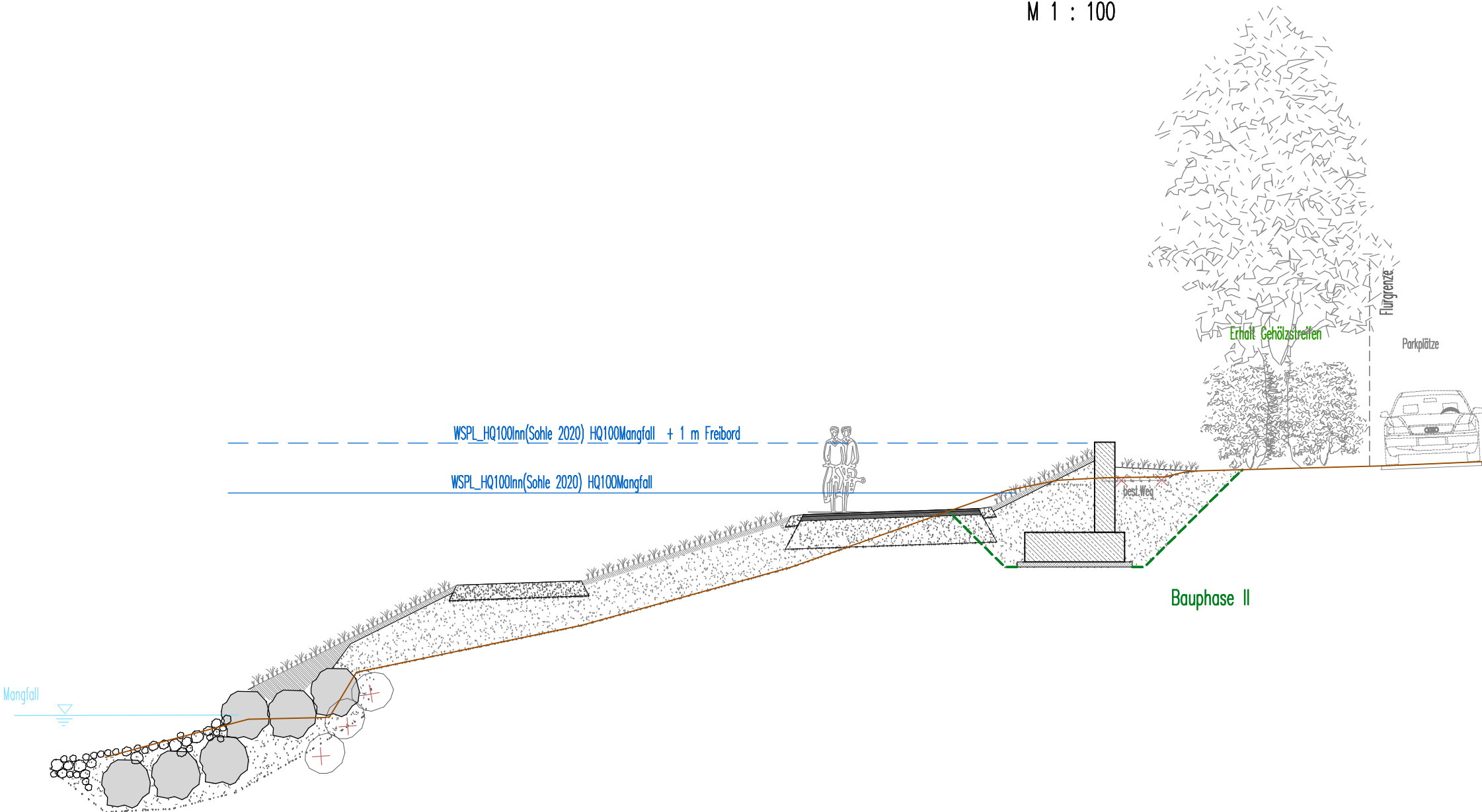
Abschnitt 1.3 Innsbrucker Str. Süd Regelquerschnitt 4.1 M 1 : 100
